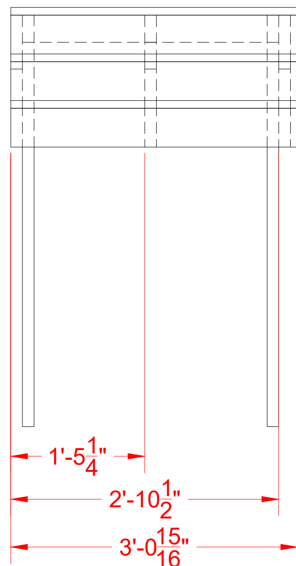
02 UPPER STAIR 101 SCALE: 1"=1'-0"
