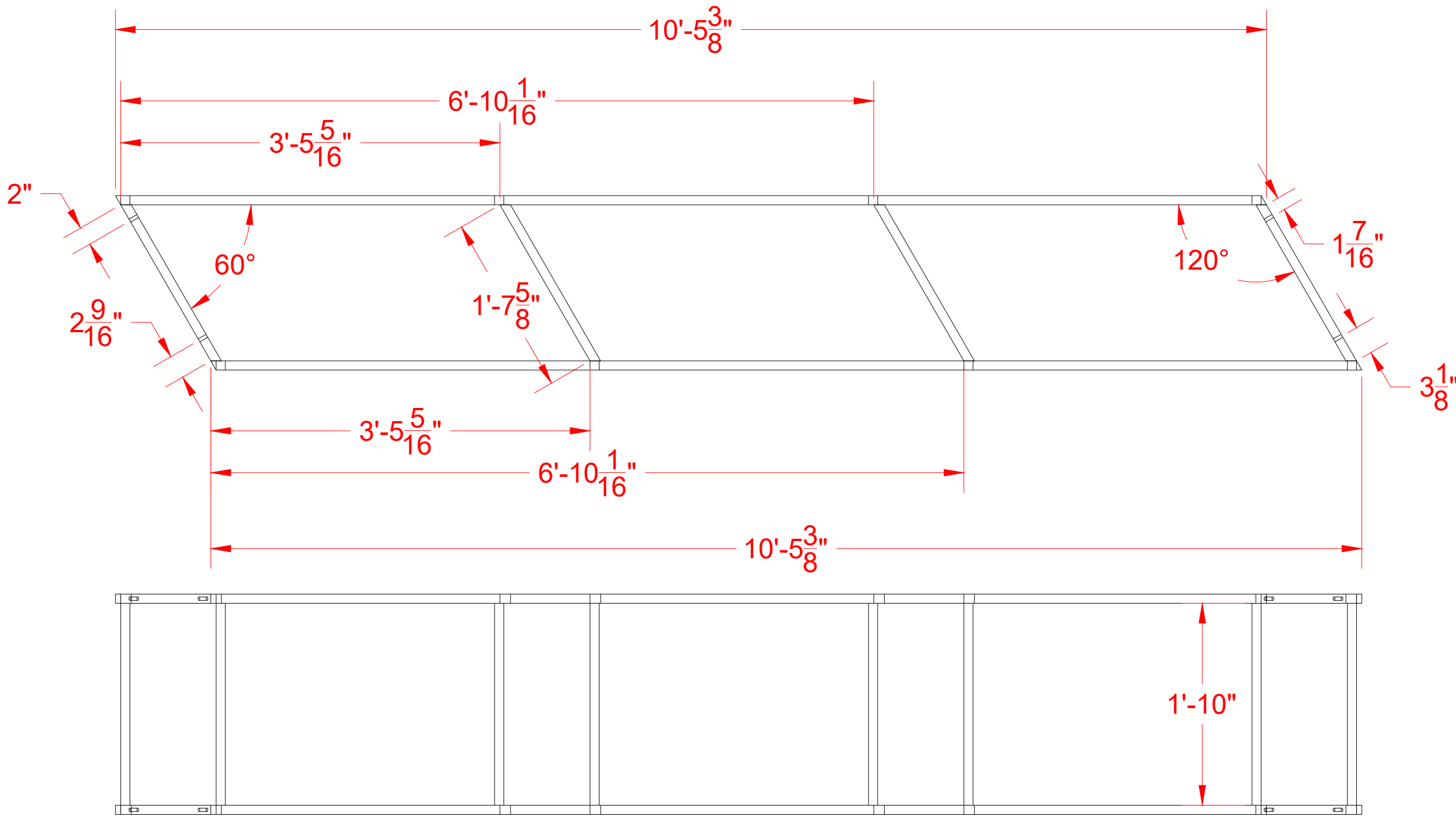
02 SECTION F 104 SCALE: 1"=1'-0"
