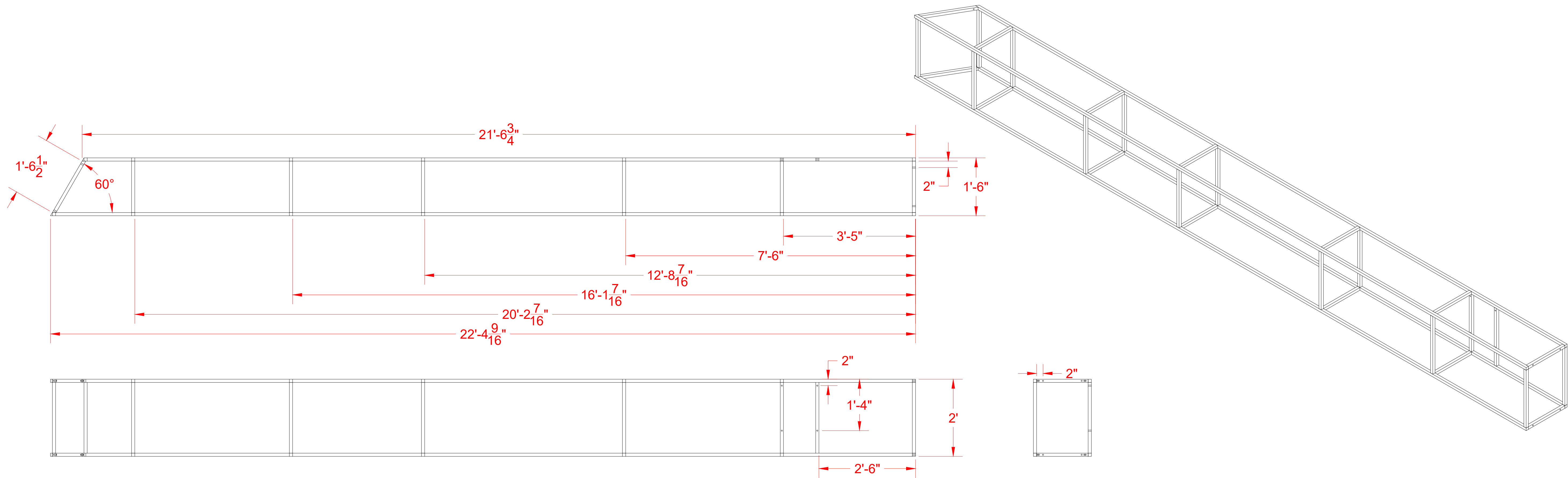
01 SECTION C 102 SCALE: 3/4" = 1'-0"
