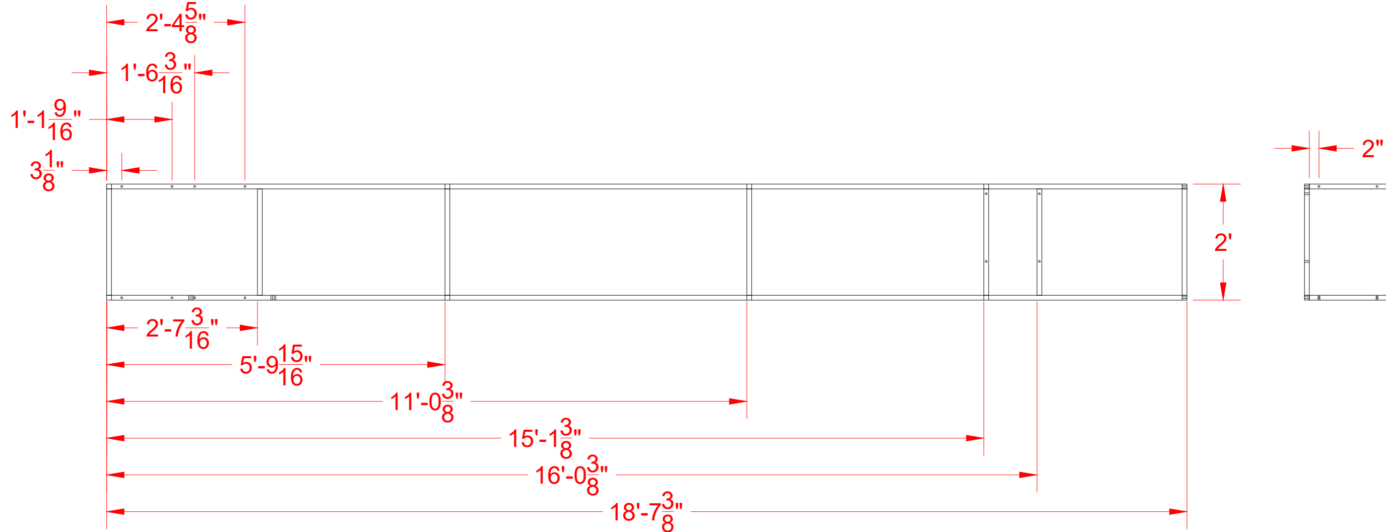
02 SECTION B SCALE: 3/4" = 1'-0"
